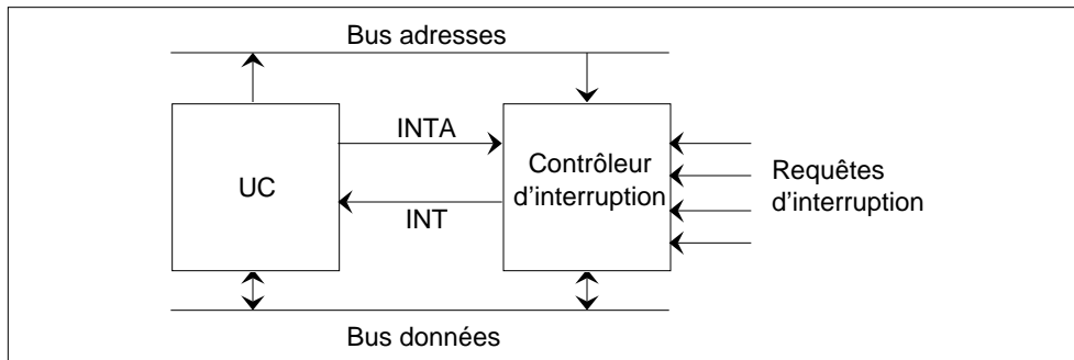
Figure 9.8: Contrôleur de priorités
