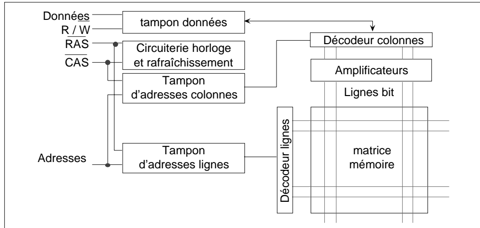
Figure 7.12: Organisation interne d'une DRAM
