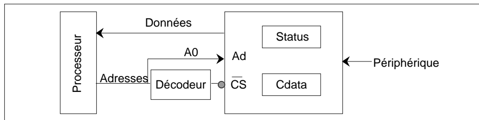
Figure 9.4: Connexion Interface-processeur
