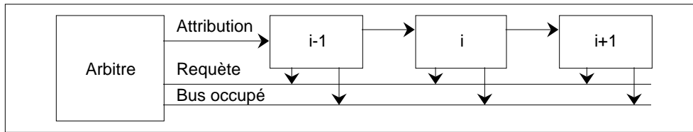
Figure 9.5: Arbitrage par chaînage
