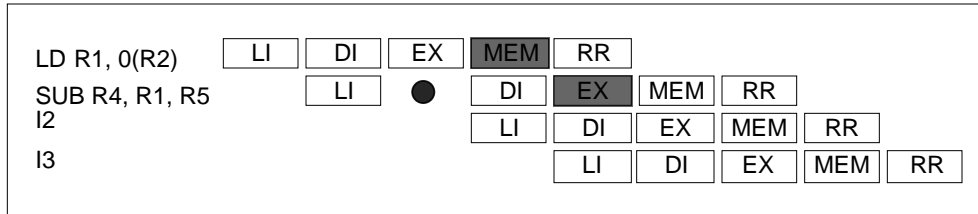
Figure 6.13: Décalage des instructions dû à une suspension
