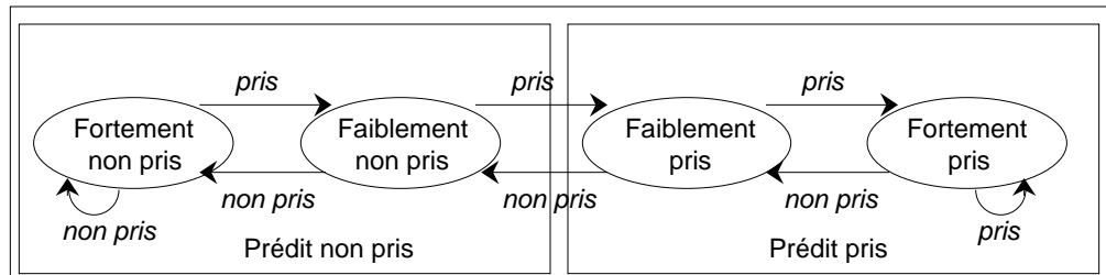
Figure 6.26: Prédicteur 2 bits
