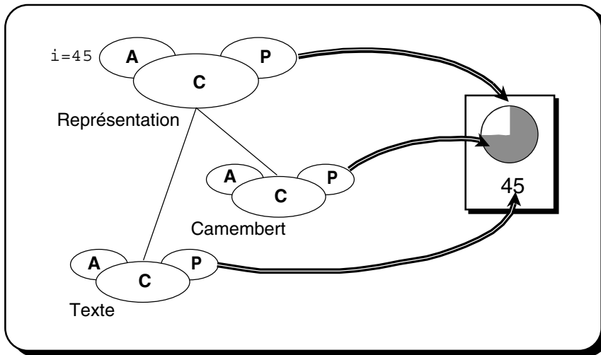
FIG. 5.4 - Utilisation du modèle PAC (Schéma de S. Chatty)
