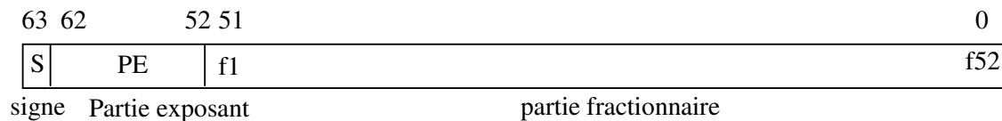
Figure 3 - Format flottant double précision.
